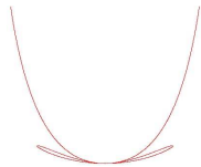
\varphi_{\vartheta}^4(\mathcal{D})
